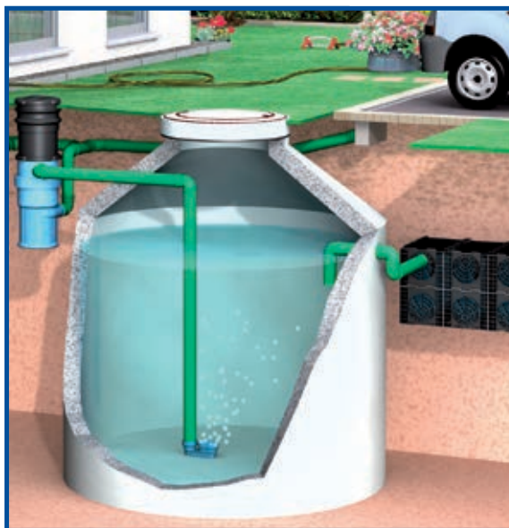
Återvinning av regnvatten. Renat vatten samlas i tank. Överflyllnadsskyddet leder det till infiltration.
