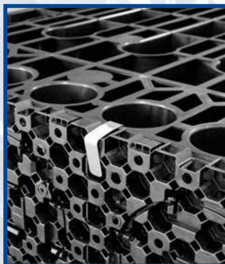
Klips för Sidoplatter. Spänns enkelt över plattan och sammanbinder denna mot kassetten.
