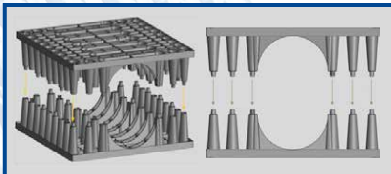
Stapla av och vänd modulen 180 grader. Tryck ihop – Klick – färdigt.
