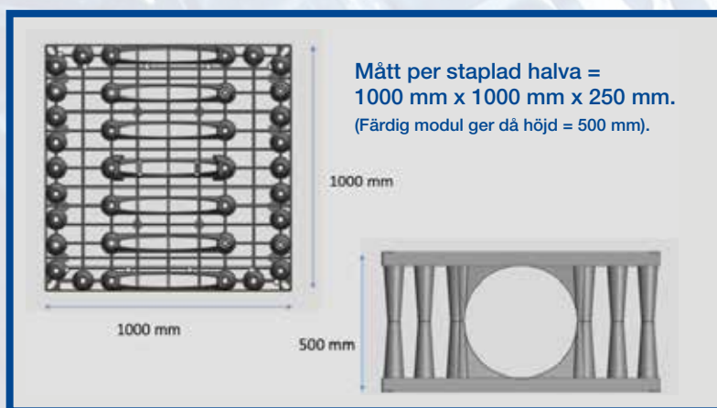
Stapla av och vänd modulen 180 grader. Tryck ihop – Klick – färdigt.
