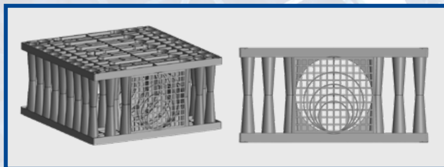
Täcklock med förmarkerade anslutningsstorlekar. Kan anslutas nedåt alt uppåt (180 grader) beroende på önskad inloppshöjd.
