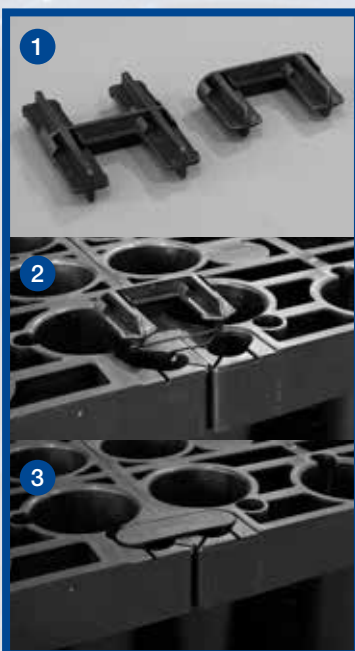
Låsplugg, Dubbel resp Enkel. För installation av kassetter i höjd resp längsled.
