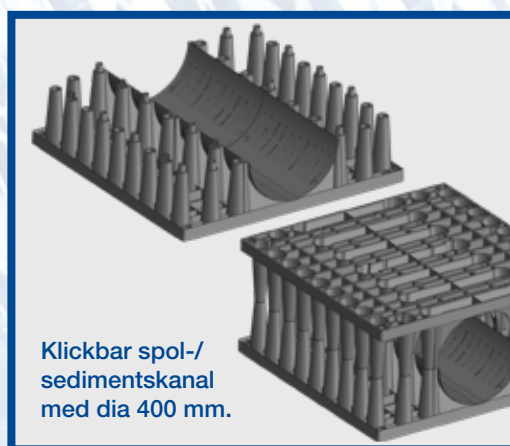
Stapla av och vänd modulen 180 grader. Tryck ihop – Klick – färdigt.
